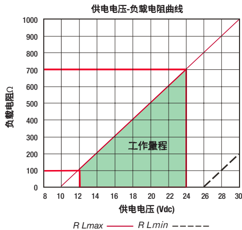
供电 - 负载电阻
