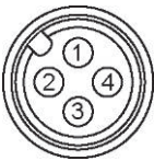
电气连接 针脚配置
